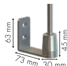
GUIDA ASTINA INOX ø10 mm
