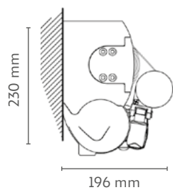
Montaje a pared
