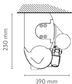
Montaje a techo
