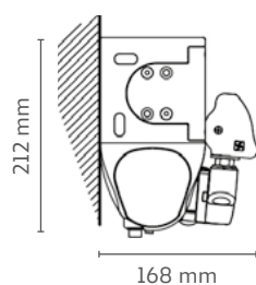
Installazione parete
