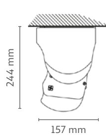
Installazione soffitto 90°
