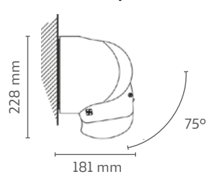
Installazione parete 75°
