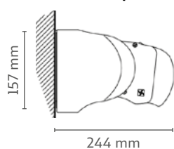
Installazione parete
