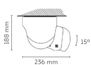
Installazione soffitto 15°
