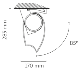
Installazione soffitto 85°
