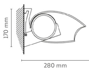
Installatione parete
