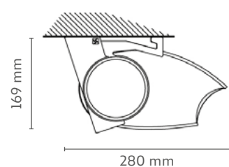
Installazione soffitto
