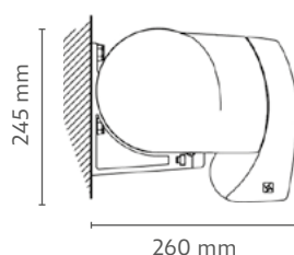
Montaggio a parete con il terminale cofre
