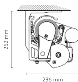
Installazione soffitto
