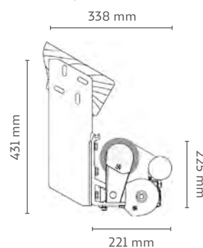
Installazione sottocoperta
