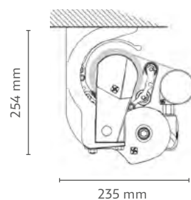
Installazione soffitto con staffe universali
